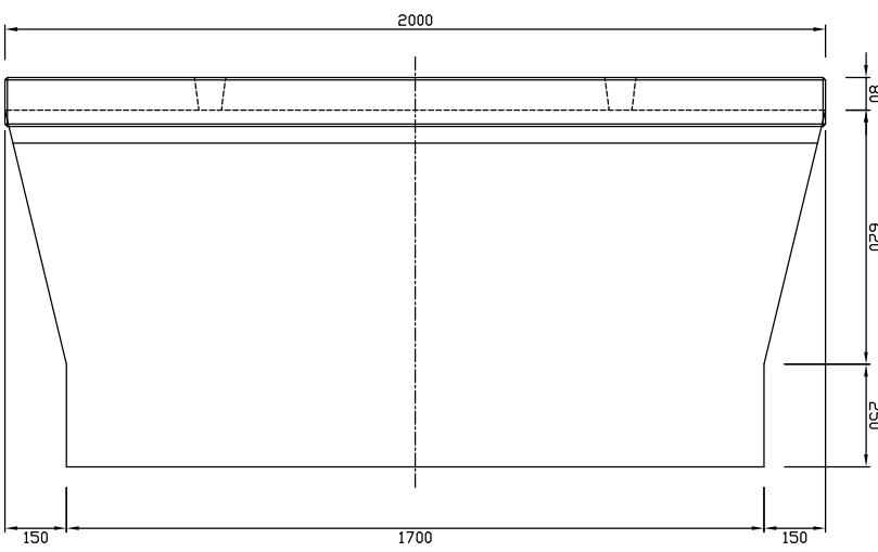
底版図
