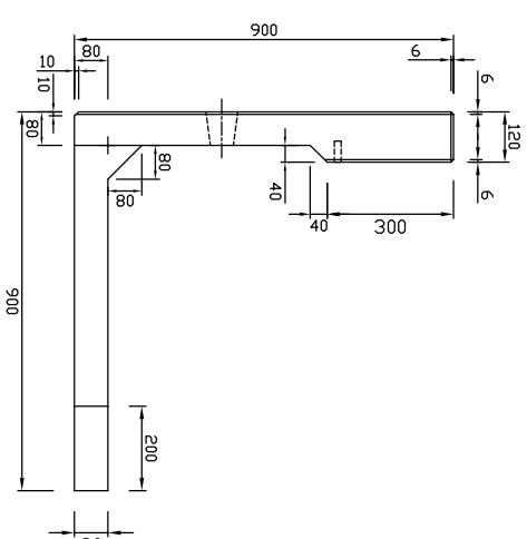
底板図
