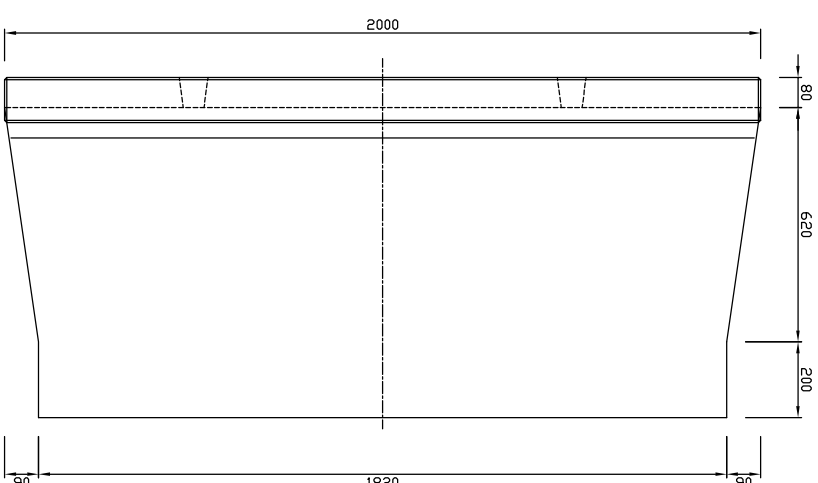
底板図
