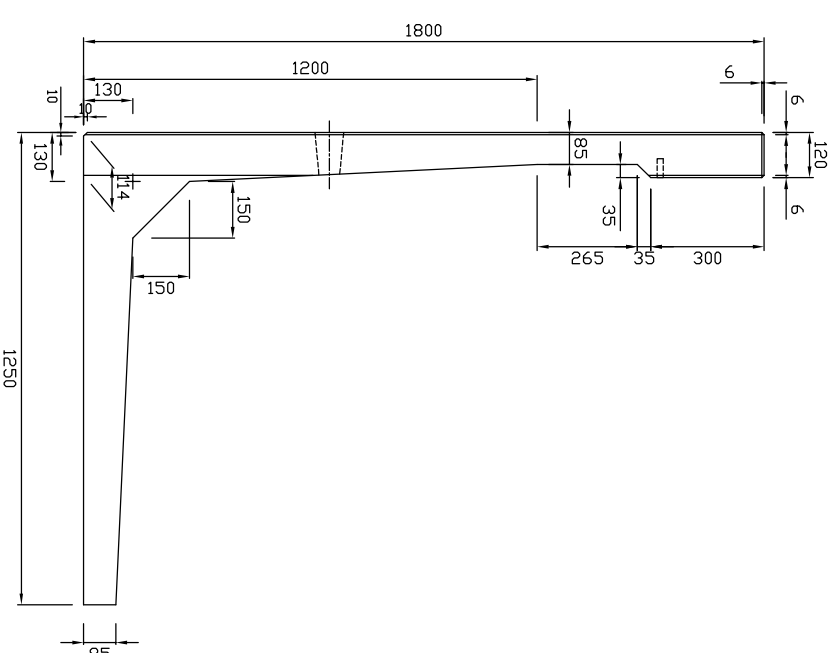
底版図
