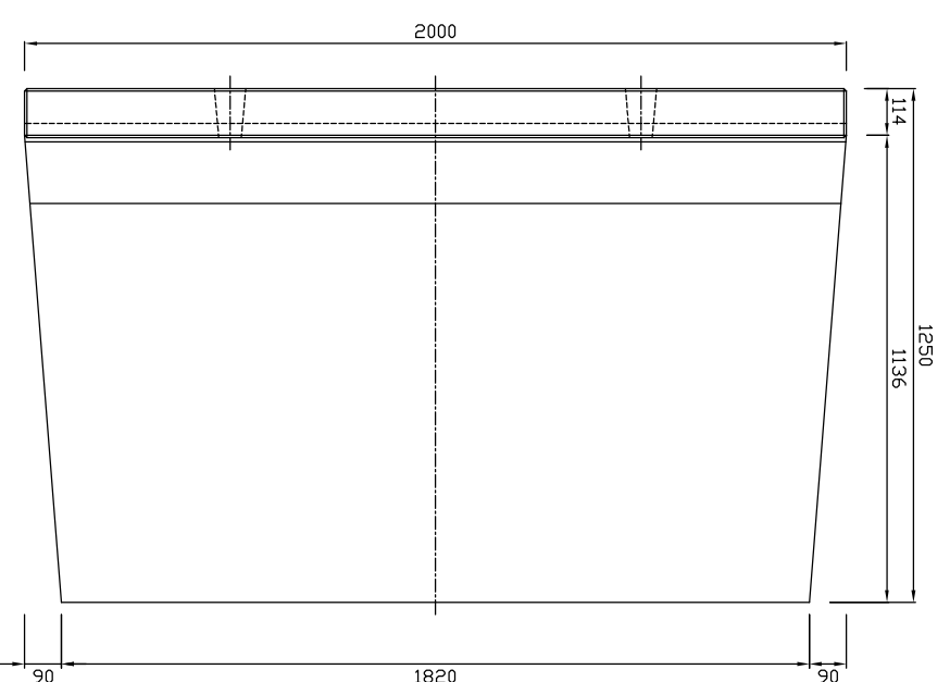
底版図
