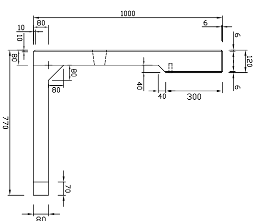
底版図
