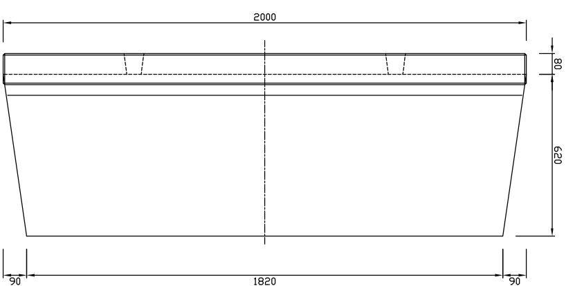
底版図
