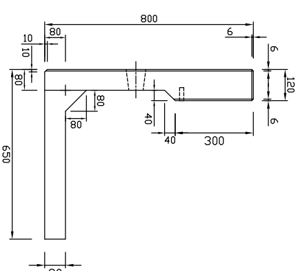
底板図
