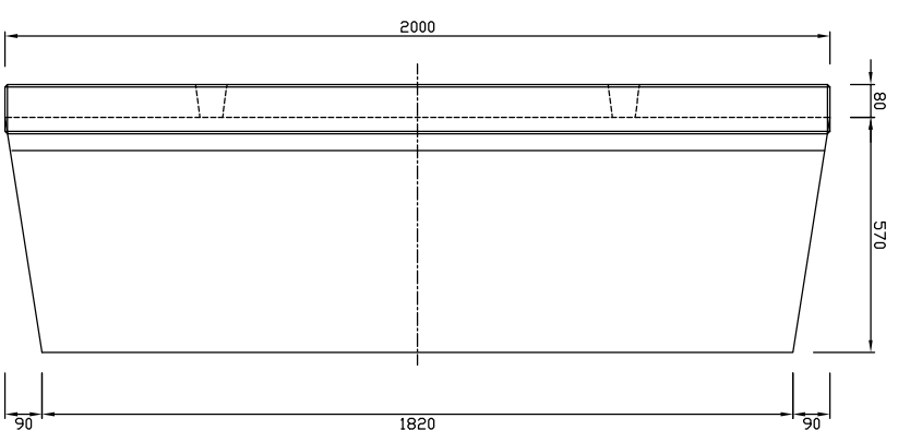
底板図
