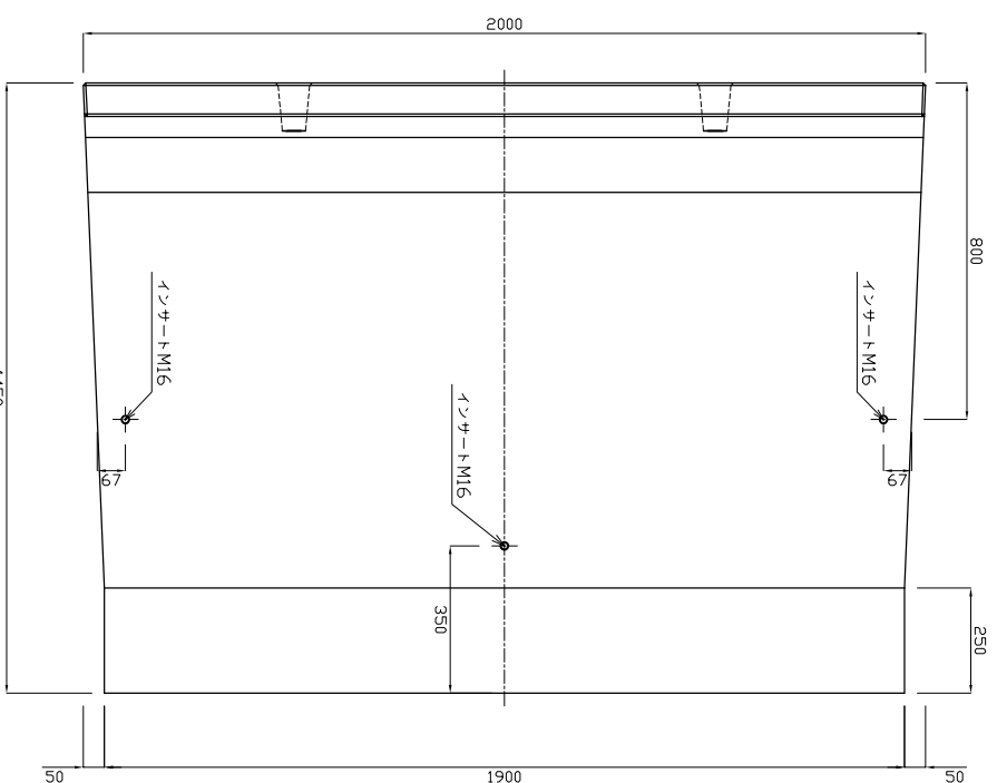
底版図
