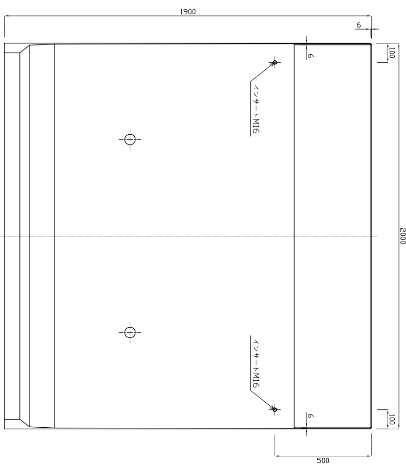
背面図
