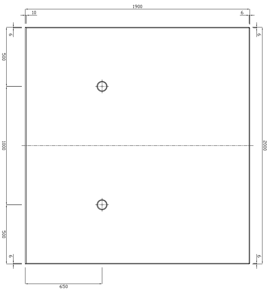
正面図
