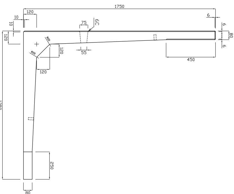
底版図
