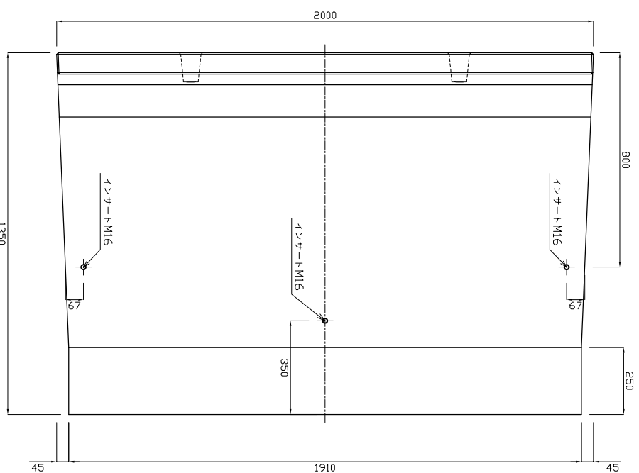
底版図
