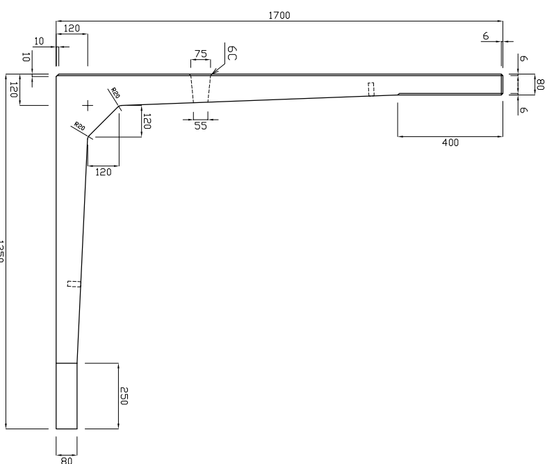
底版図
