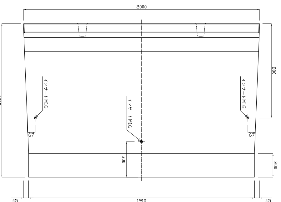
底版図
