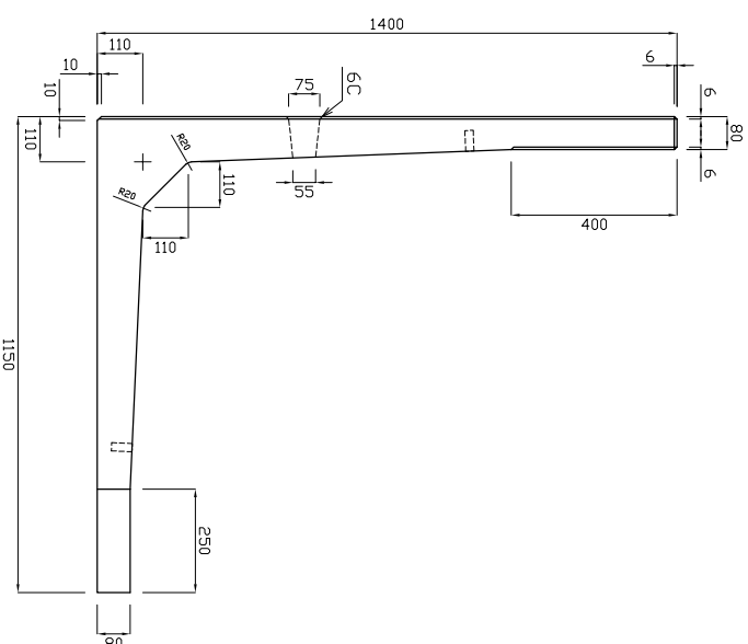
底版図
