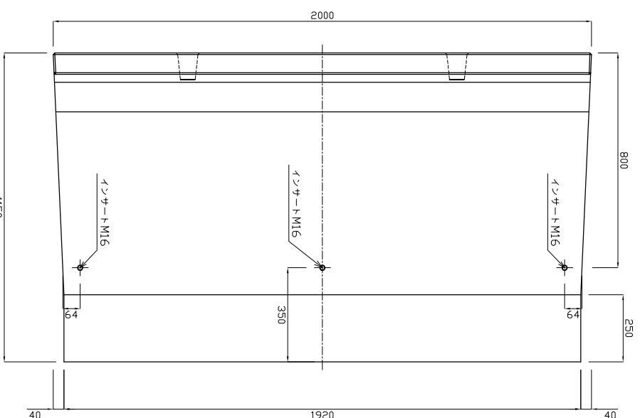
底版図
