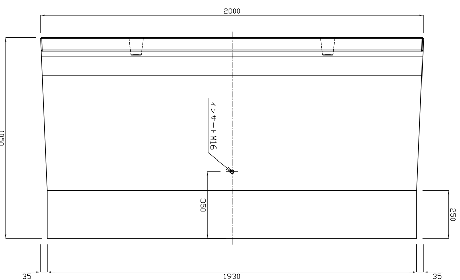
底版図
