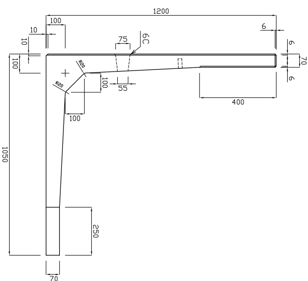
底版図
