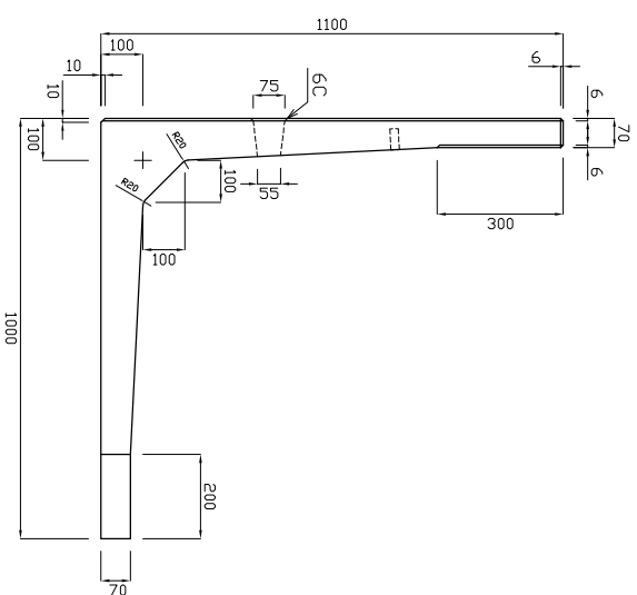
底版図
