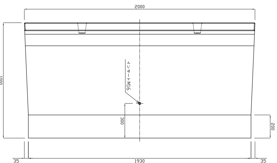
底版図
