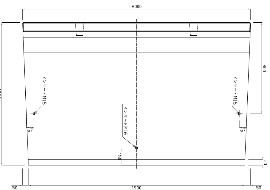
底版図
