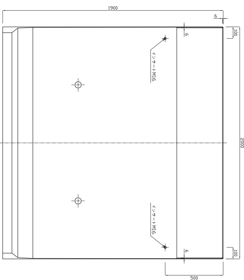
背面図
