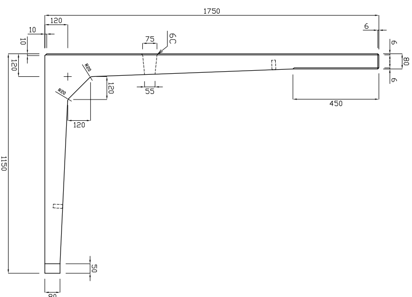
底版図
