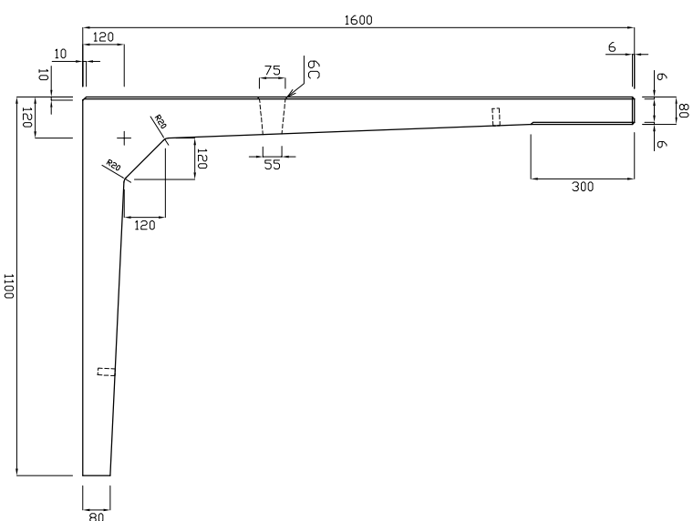
底版図
