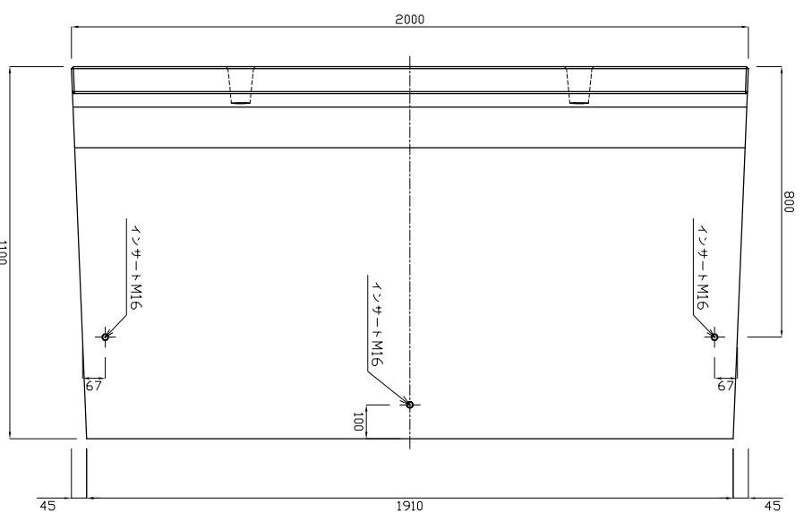
底版図
