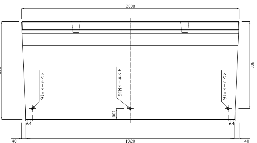
底版図
