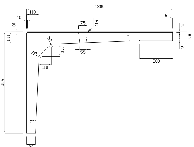
底版図
