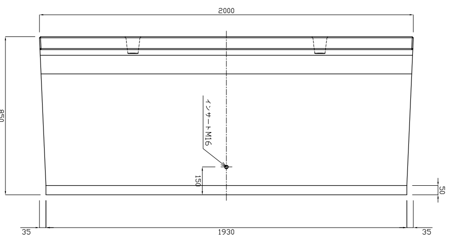
底版図
