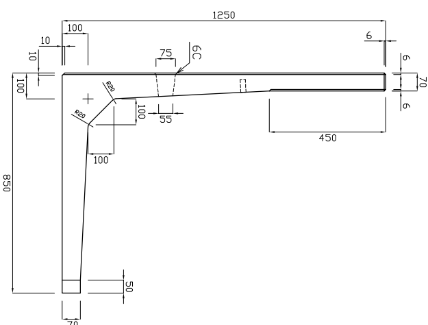
底版図
