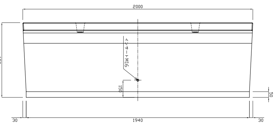
底版図
