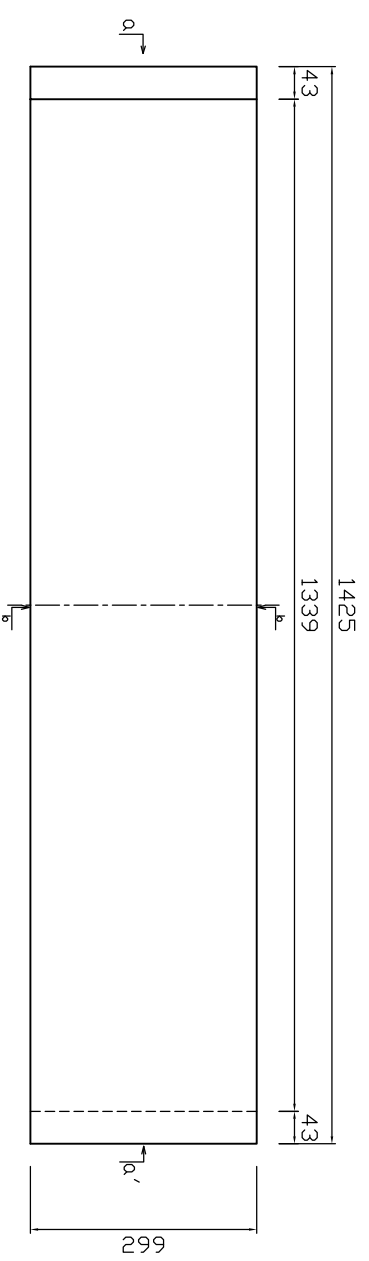
正面図
